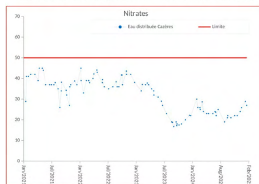
Courbe d'évolution de la concentration en nitrates (mg/l) depuis 2021 :
